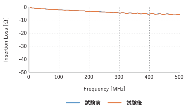
Insertion Loss測定結果
